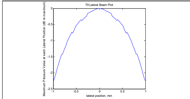
Fig.(d) TX Lateral beam-plot
